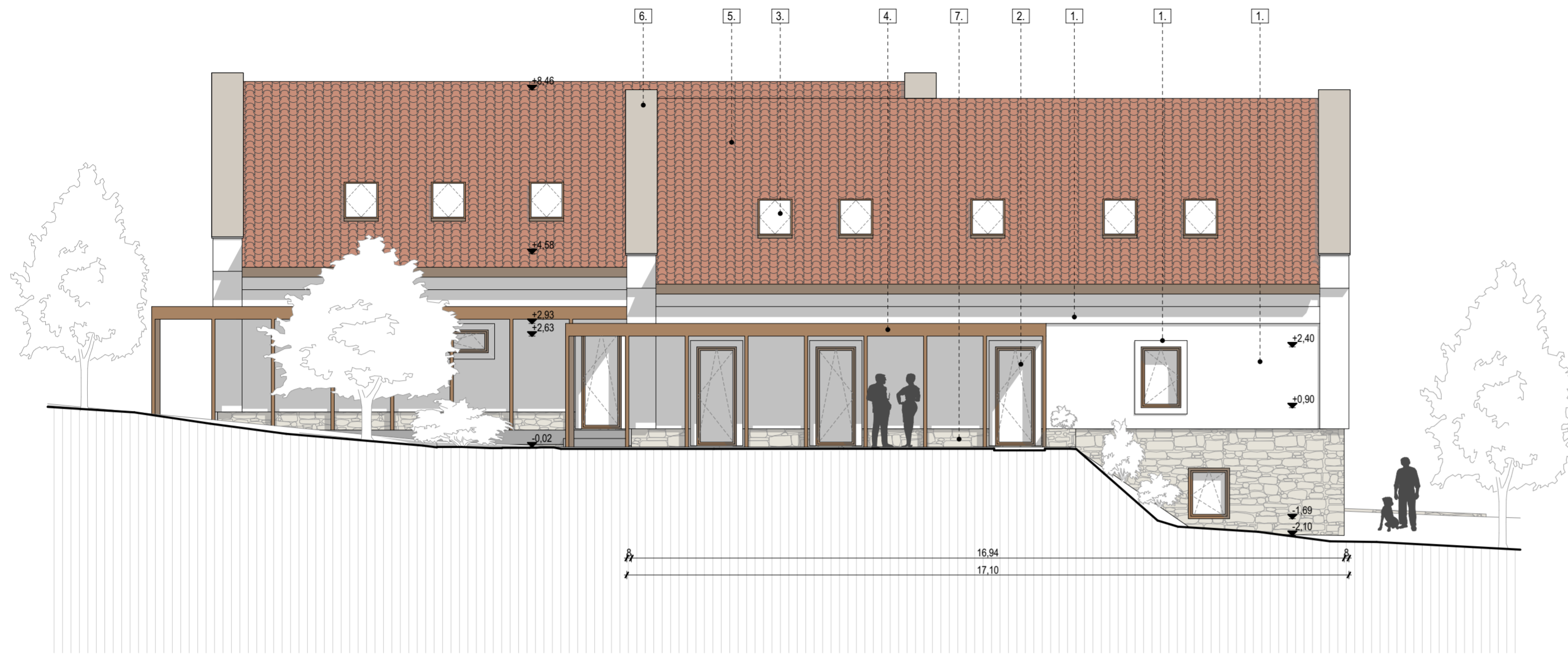
NYUGATI HOMLOKZAT M 1:100
